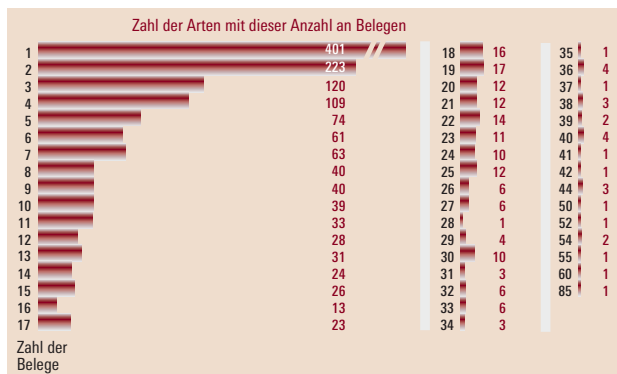
Abb. 3 Anzahl der Arten mit einer bestimmten Anzahl von Herbarbelegen.
